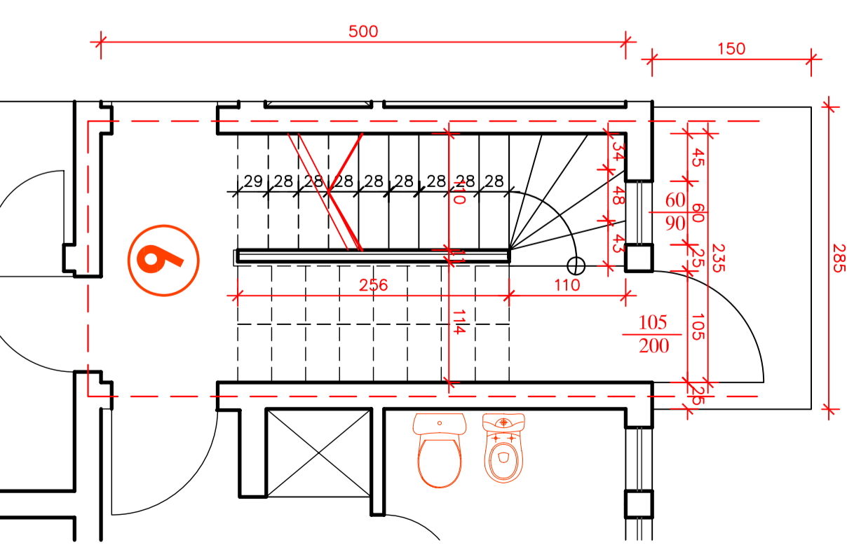
ДЕТАЙЛ ВХОД КОТА + 0,00 М 1:50 ст. клетка 13,8м 2 бруто площ
